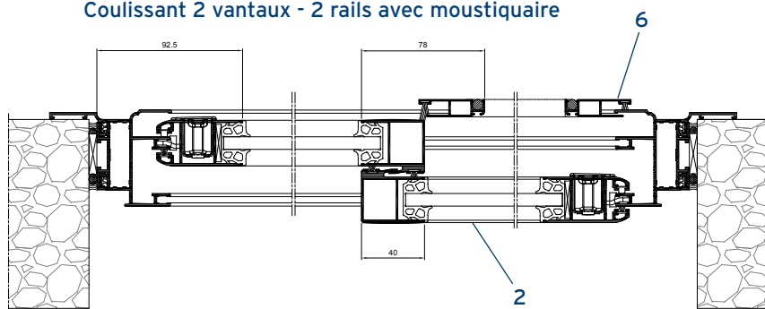
Coulissant 2 vantaux - 2 rails avec moustiquaire
