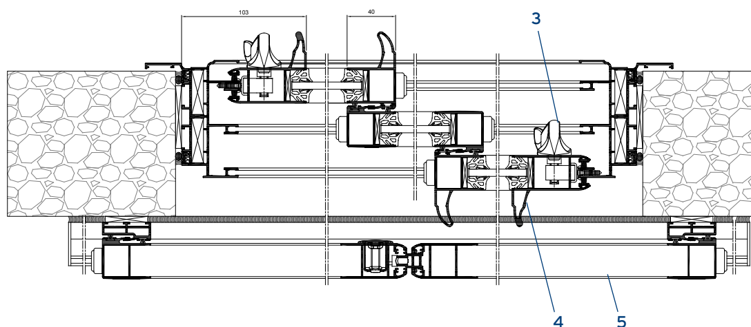
Coulissant 3 vantaux - 3 rails avec volets coulissants
